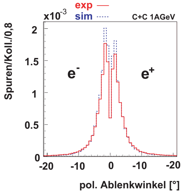
Abbildung 4.9: Verteilung der Ablenkungswinkel in polarer Richtung zwischen den vorderen Driftkammern und den META-Detektoren. Aufgetragen ist die gemessene Anzahl von Spuren pro C+C-Kollision in Schritten von 0,8^\circ . Die Akzeptanz für Elektronen ist etwas höher als für Positronen.
