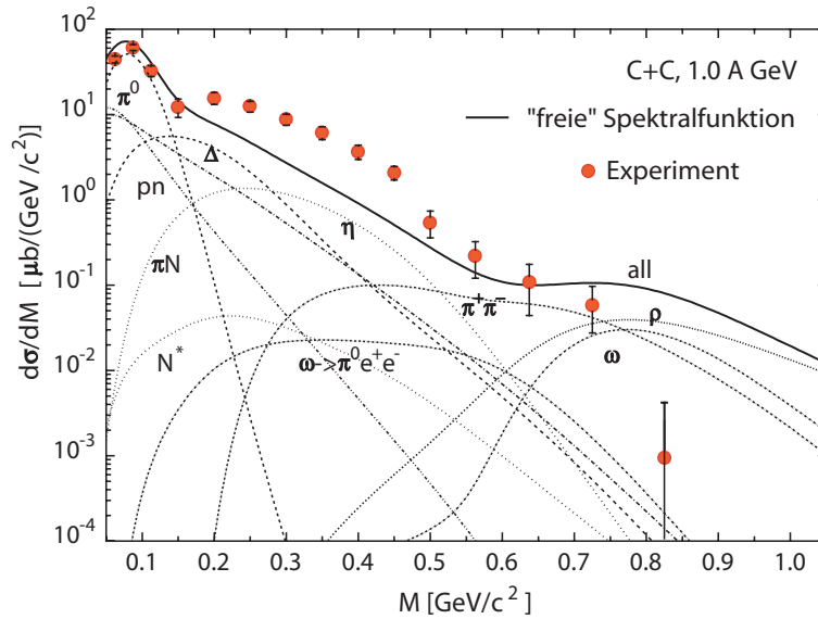
Abbildung 1.1: Von der DLS Kollaboration gemessenes invariantes Massenspektrum von e^+e^- -Paaren für die Reaktion C+C bei E = 1 \text{ GeV}\cdot\text{A} [Bra98]. Die Massenaufösung ist nicht ausreichend, um die Beiträge der verschiedenen Kanäle zu trennen.
